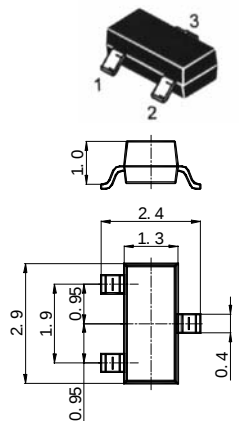
SOT-23
