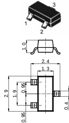
SOT-23
