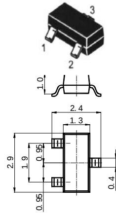
SOT-23
