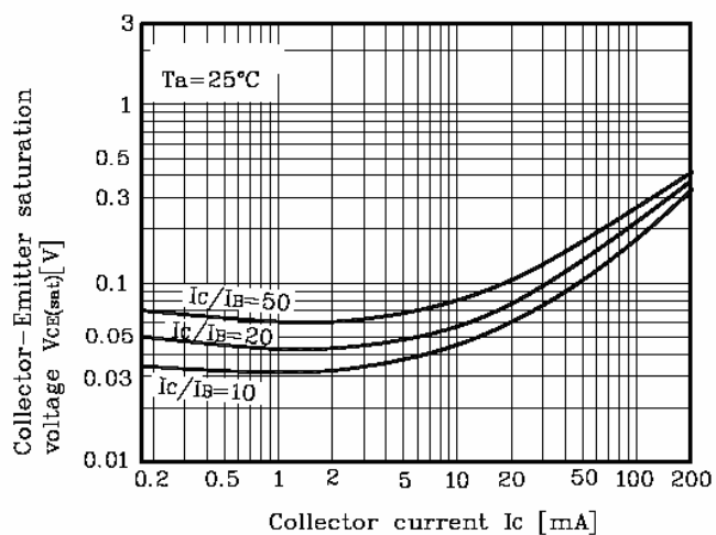
Fig. 5 V_{CE(sat)} - I_C
