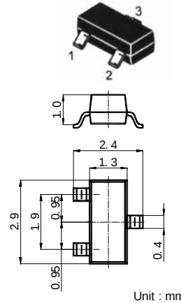
SOT-23
